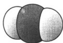
二氧化碳
