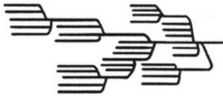
支链淀粉
