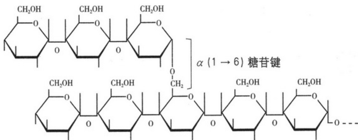
支链淀粉
