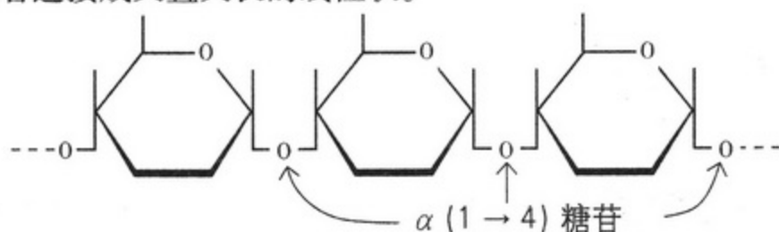
直链淀粉
