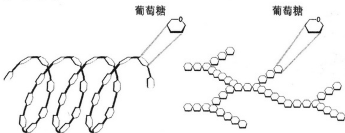
直链淀粉的结构
